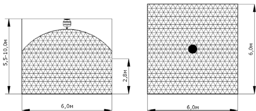
Рис.3 Масштабное изображение конфигурации распыла огнетушащего порошка.
