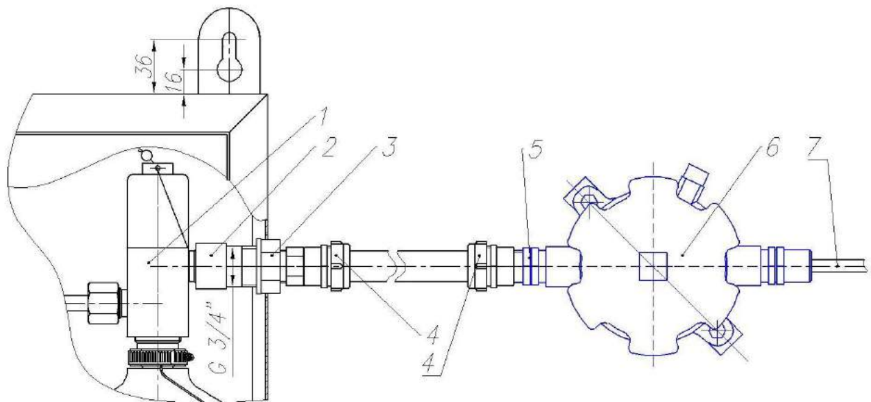
Рисунок П.3.2 Подключение модуля через взрывозащищённую коробку коммутации. 1. Запорно-пусковое устройство; 2. Переходник крепления устройства электропуска УП-ЗМ; 3. Переходник 3/4"x1/2" вн. -нар; 4. Резьбовой крепёжный элемент РКВ-20; 5. Кабельный ввод; 6. Коробка коммутации; 7. Кабель к системе автоматики. Детали поз.3-7, поставляются по заказу за отдельную плату.
