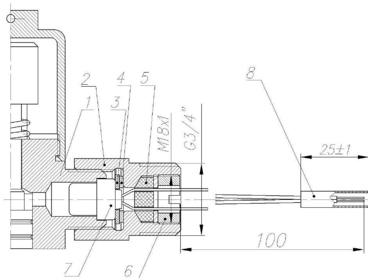
Рисунок П.3.3 Узел подключения модуля общепромышленного исполнения. 1. Запорно-пусковое устройство; 2. Переходник; 3. Прокладка паронитовая; 4. Шайба; 5. Уплотнитель резиновый; 6. Прижим; 7. Устройство электропуска УП-3М; 8. Изолирующая трубка.
