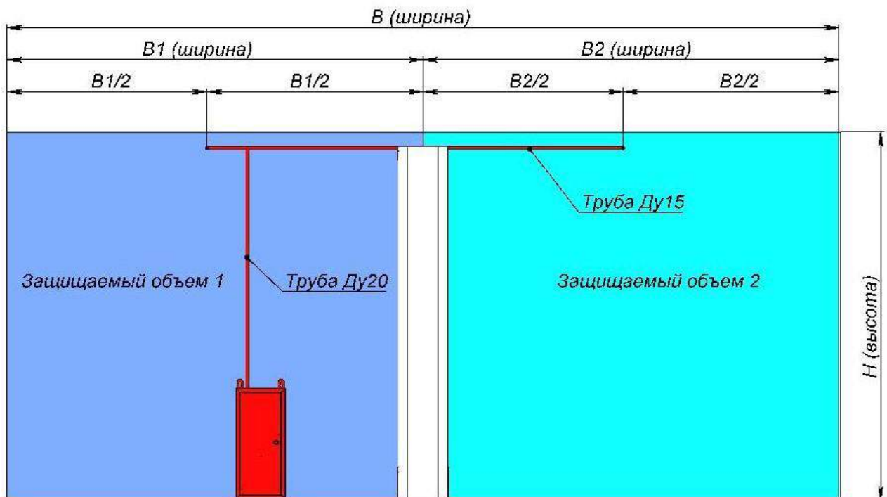
Рисунок П.1.4. Схема распыления ГПОВ при объемном тушении межстеллажного пространства двумя насадками Ду15. Вид спереди.
