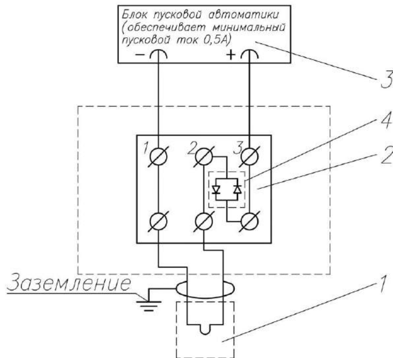
Рисунок 3. Схема подключения модуля.
