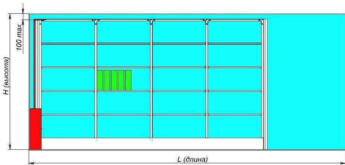
Рисунок П.1.3. Схема распыления ГПОВ при объемном тушении межстеллажного пространства двумя насадками Ду15. Вид сбоку.
