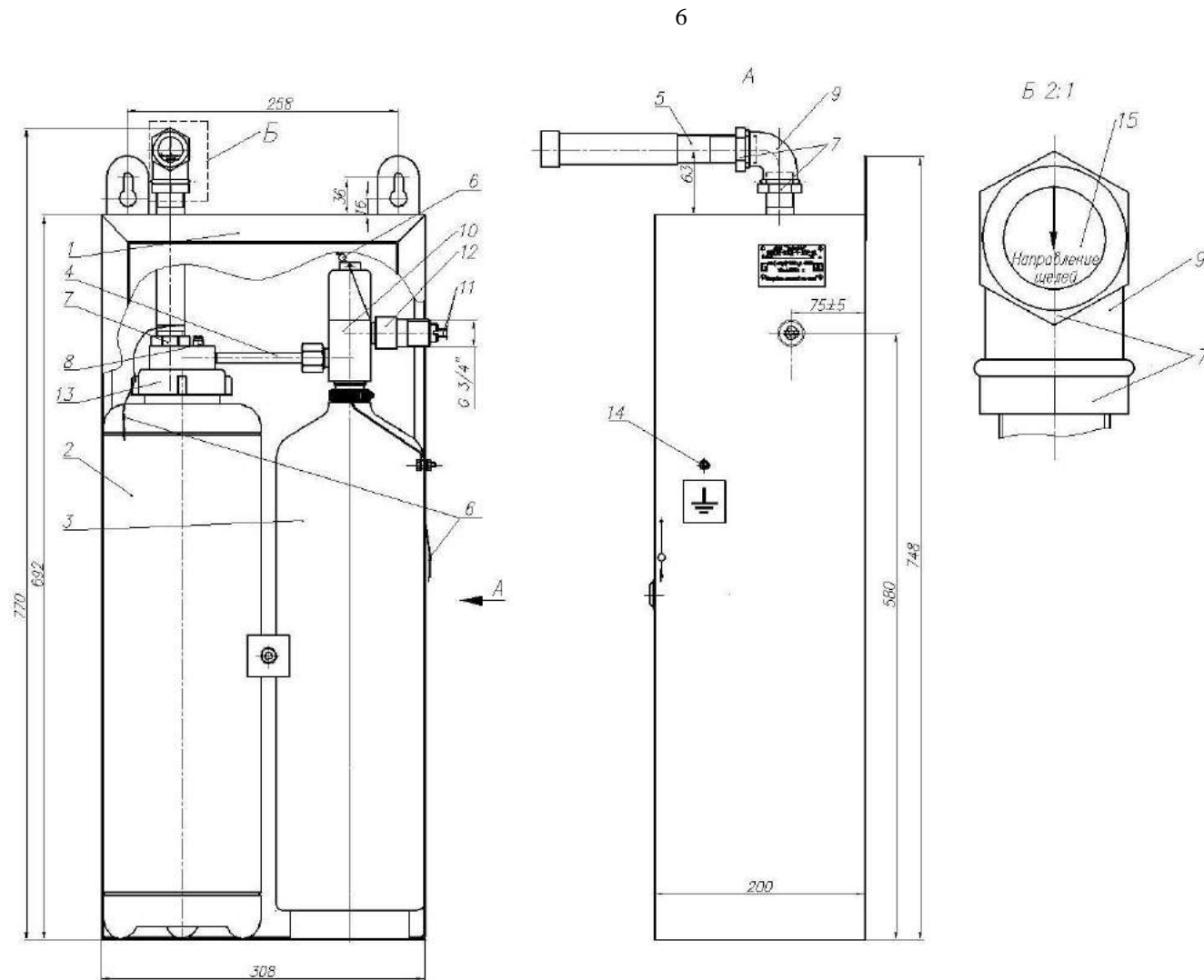
Рисунок 1. Устройство модуля
