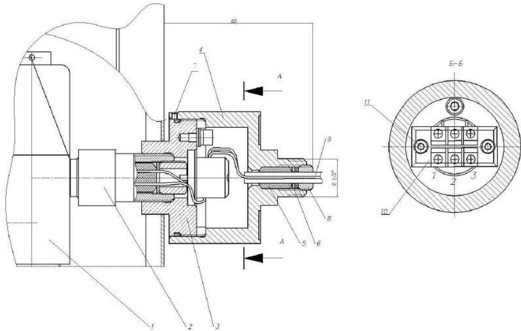
Рисунок П.3.1 Подключение модуля через коробку коммутации находящуюся на модуле. 1. Запорно-пусковое устройство; 2. Переходник крепления устройства электропуска УП-ЗМ; 3. Корпус; 4. Крышка; 5 Уплотнитель резиновый, d_{вн} = 6 и 8мм; 6. Шайба стальная; 7. Стопорный винт; 8. Прижим; 9. Кабель от системы автоматики диаметром от 4 до 8мм; 10. Клеммная колодка ТВ-1503; 11. Винт.
