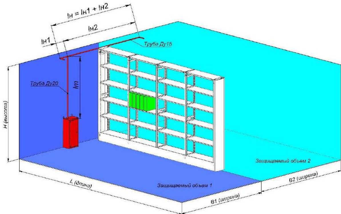
Рисунок П.1.2. Схема распыления ГПОВ при объёмном тушении межстеллажного пространства двумя насадками Ду15
