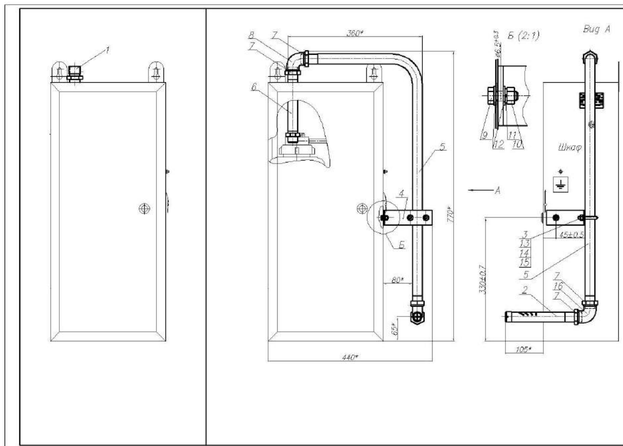
Рисунок П.4.7. Модуль с нижней разводкой насадка
