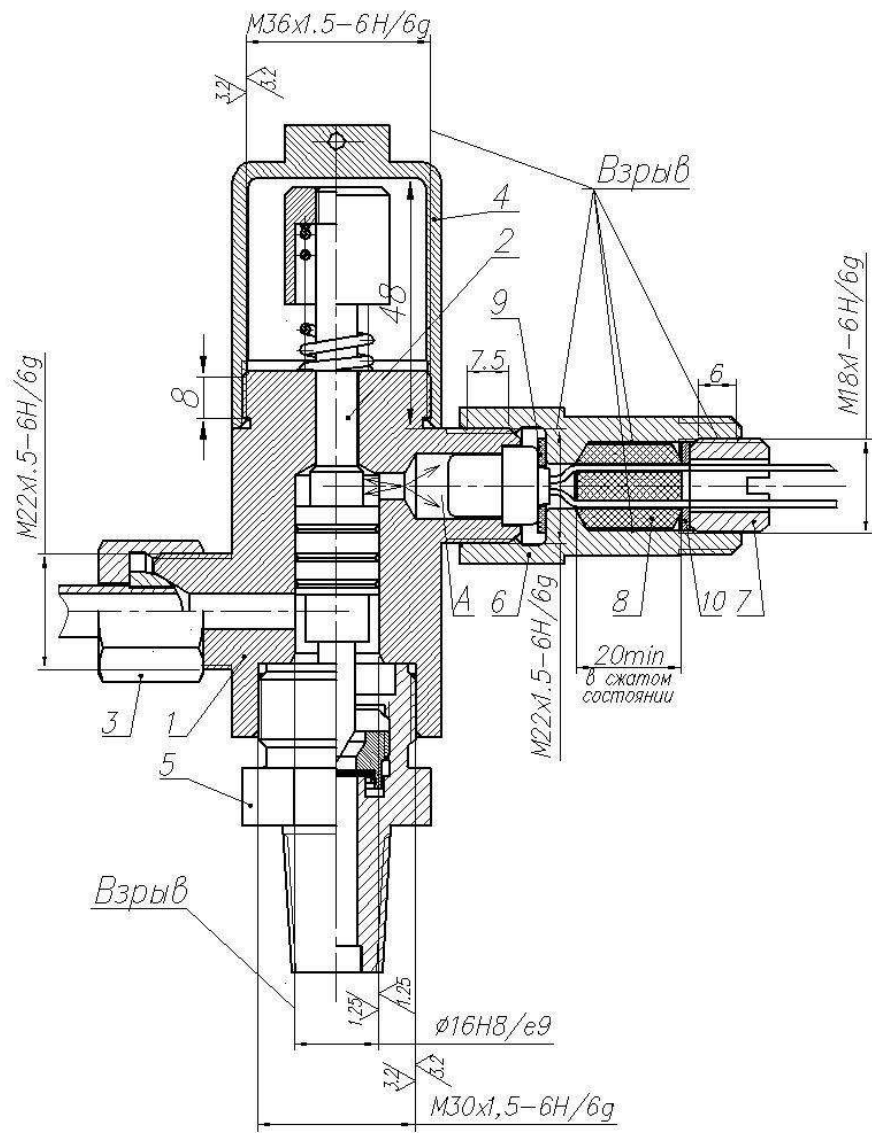
Рисунок 2. Средства взрывозащиты запорно-пускового устройства модуля МПП(Н)-8-КД-1-БСГ-У2.
