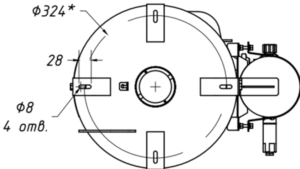
Рисунок 9. Места крепления МПП «Гарант-100вз».
