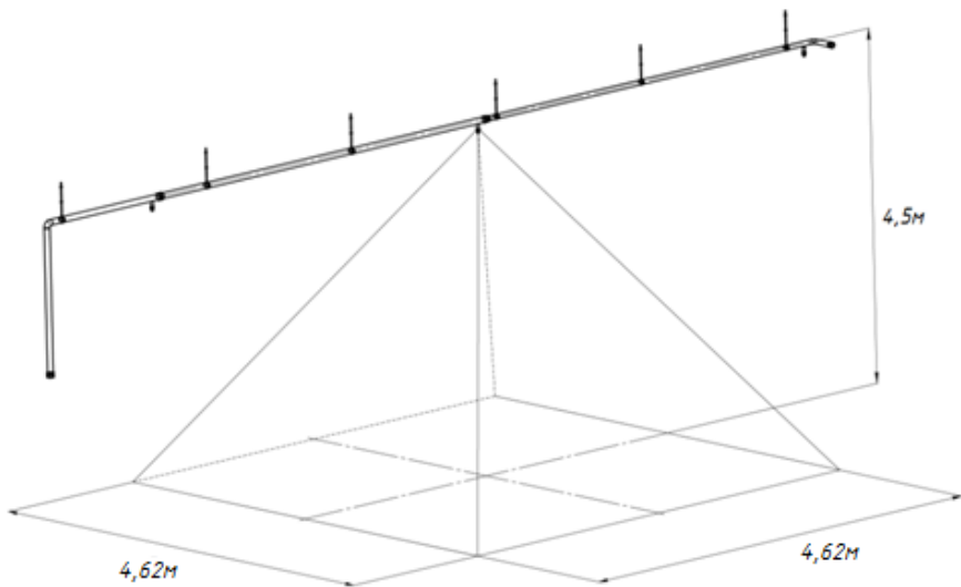
Рисунок 4а. Конфигурация диаграммы распыления порошка с применением насадка-распылителя «РП-20».
