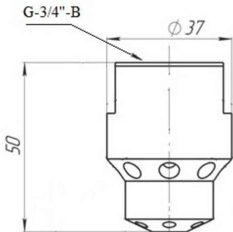
Рисунок 6. Насадок-распылитель «РП-20».
