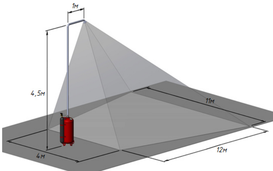
Рисунок 3. Конфигурация диаграммы распыления порошка с применением насадка-распылителя «РП-50», направленного под углом 45о к горизонтальной поверхности.
