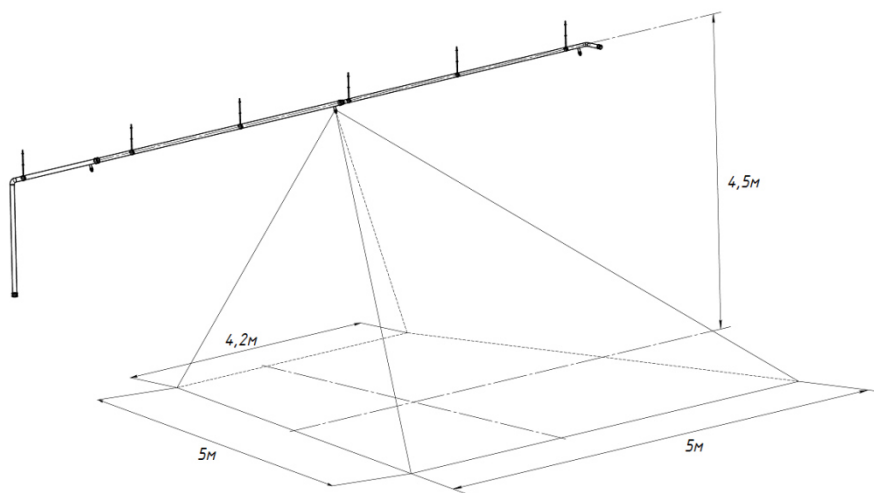
Рисунок 4б. Конфигурация диаграммы распыления порошка с применением насадка-распылителя «РП-20», направленного под углом 45° к горизонтальной поверхности.
