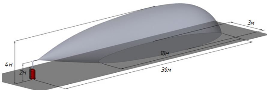
Рисунок 2. Конфигурация диаграммы распыления порошка без применения насадка-распылителя.
