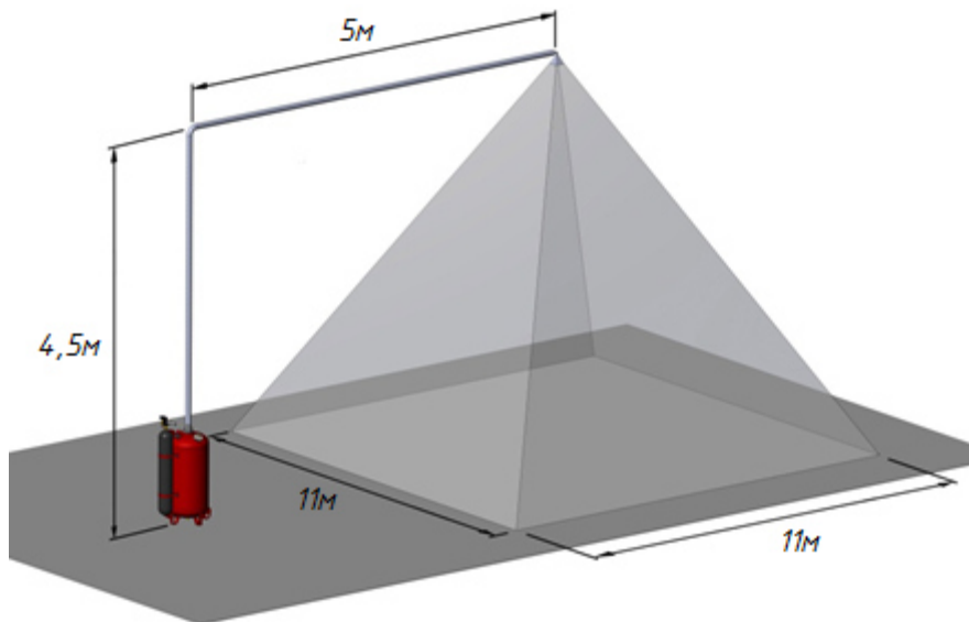
Рисунок 1. Конфигурация диаграммы распыления порошка с применением насадка-распылителя «РП-50».
