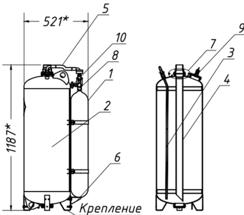
Рисунок 5. Конструкция МПП «Гарант-100вз».
