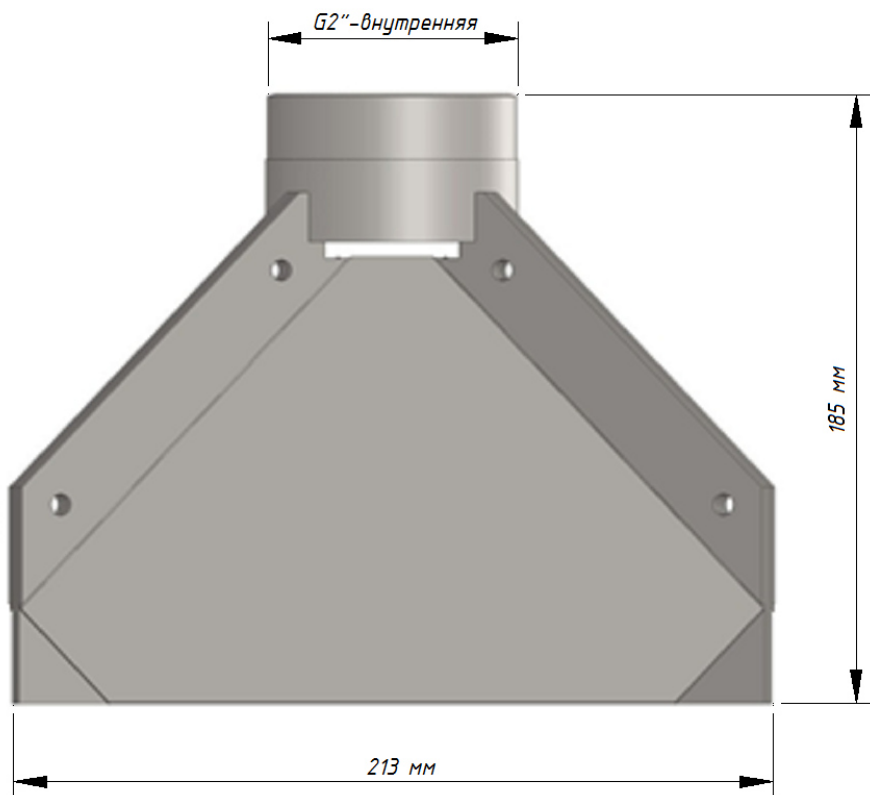
Рисунок 7. Насадок-распылитель «РП-50».
