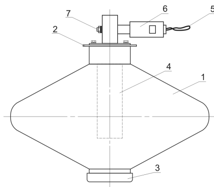
Рис. 2 – Конструкция МПП «Гарант-12-ВЗ».
