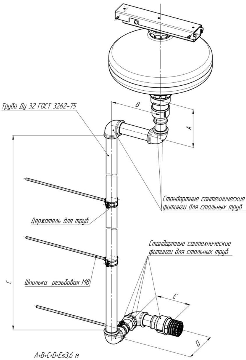
Рис. 4. Общий вид модуля МУПТВ-14,5-ГЗ-ВД во взрывозащищенном исполнении с удлиненным трубопроводом Ду32.
