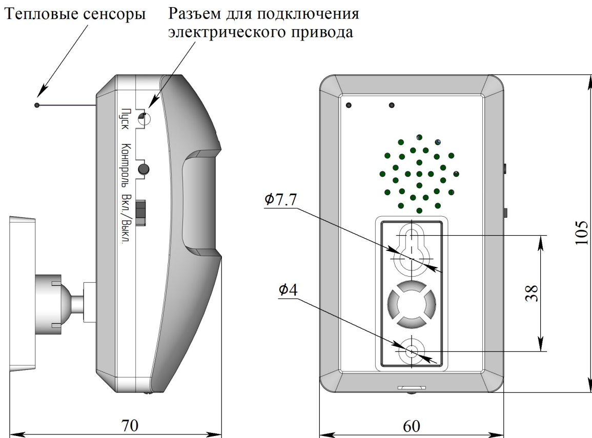
Рисунок 2 – Внешний вид устройства
