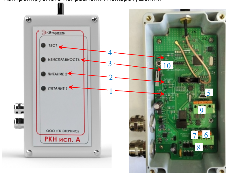
Рисунок 4.5 Внешний вид радио контроллера направления (РКН) исп. А. с установленной и снятой лицевой панелью.
