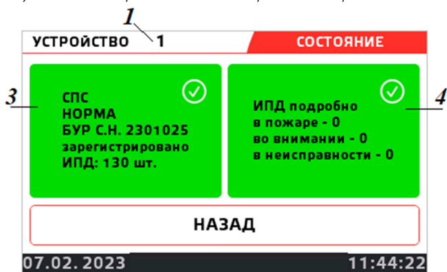
Рисунок 4.17.б. Экран состояния выбранного направления СПС.
