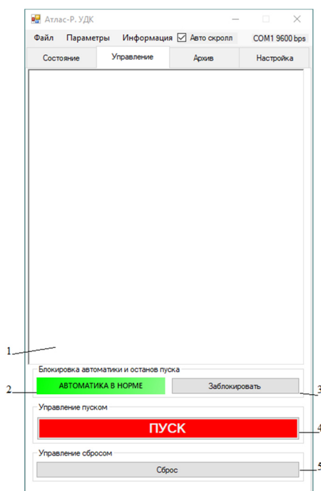
Рисунок 5.4 Внешний вид рабочей области «Управление».
