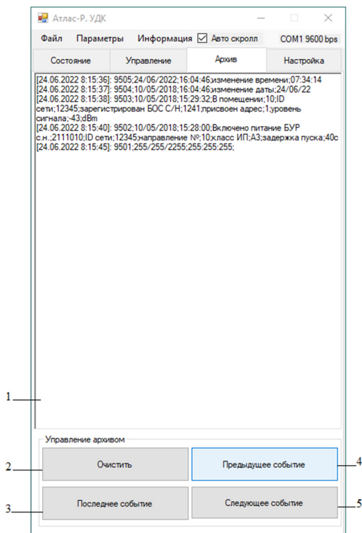
Рисунок 5.5 Внешний вид рабочей области «Архив».
