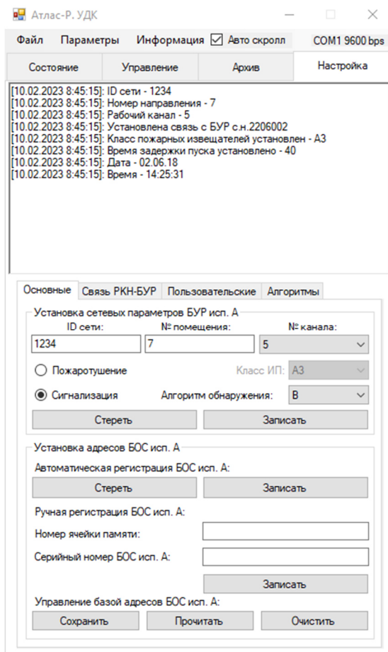
Рисунок 5.6. Внешний вид рабочей области «Настройка».
