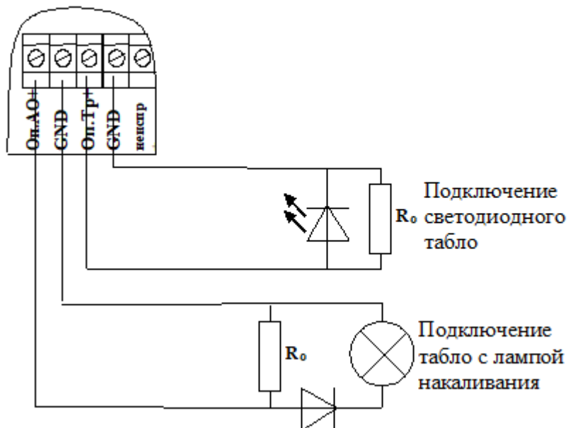
Рисунок Пб.1. Схема подключения шлейфа сигнализации датчиков контроля закрытия дверей к БУР исп. А.
