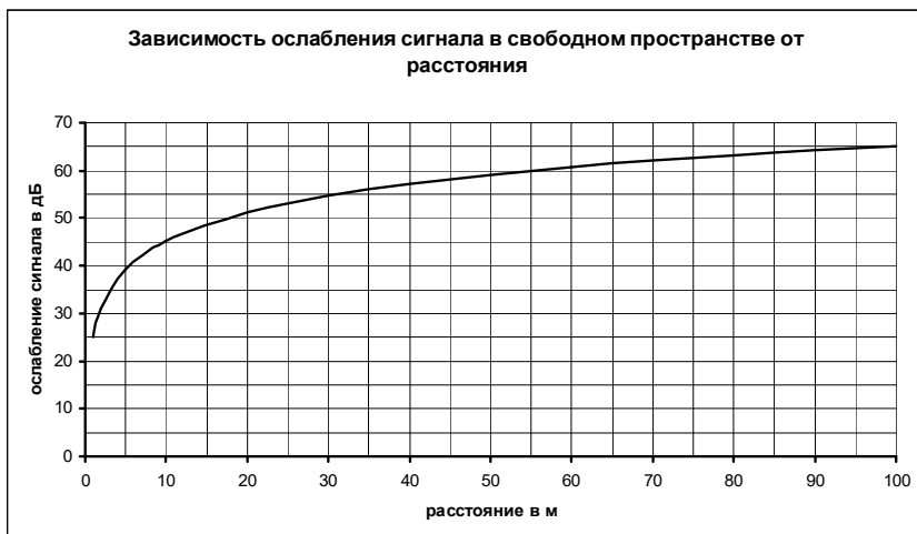
Рисунок 6.1. Ослабление сигнала на радиолиниях в свободном пространстве.
