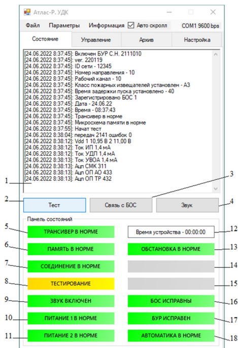
Рисунок 5.3 Внешний вид рабочей области «Состояние».
