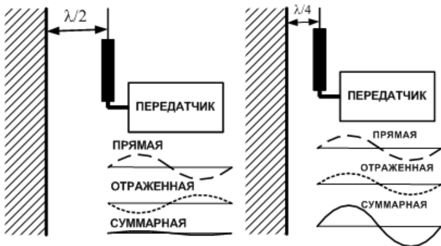
Рисунок 6.2. Размещение антенны БУР исп. А в непосредственной близости от стены.
