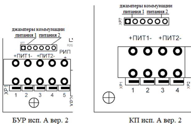
Рисунок П1.2. Расположение клемм подключения и джамперов коммутации питания БУР, КП (версия 2).
