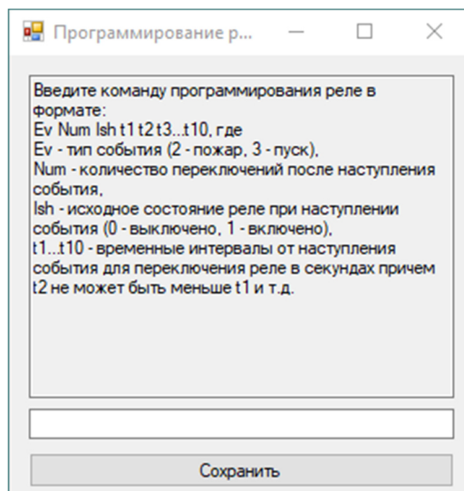
Рисунок 5.8. Внешний вид окна программирования реле.
