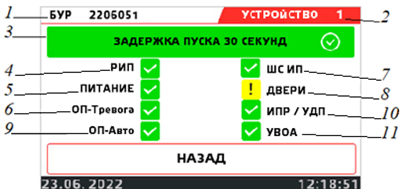
Рисунок 4.18. Экран подробной информации о состоянии БУР / РКН исп. А.
