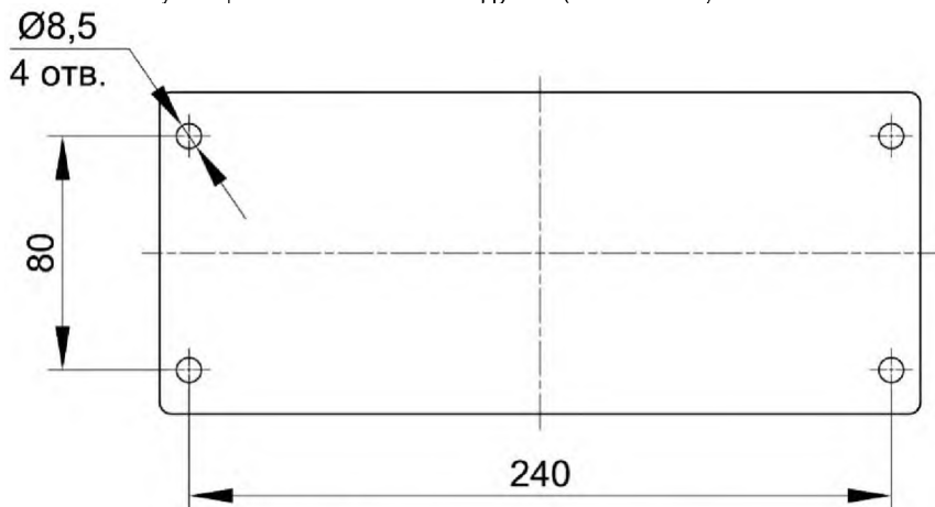
Рисунок 4 - Координаты крепления модуля.
