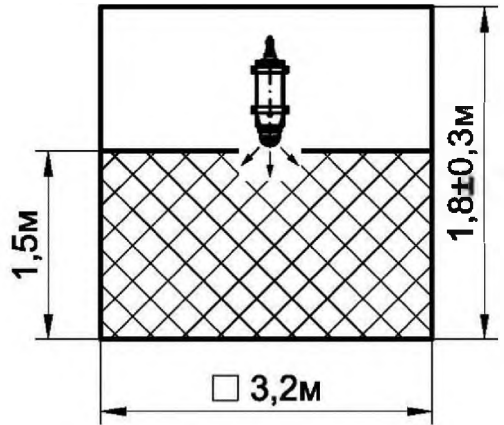
Рисунок 8 - Масштабное изображение области, в которой достигаются условия тушения модулем Буран-2,0(1) по очагам класса А.
