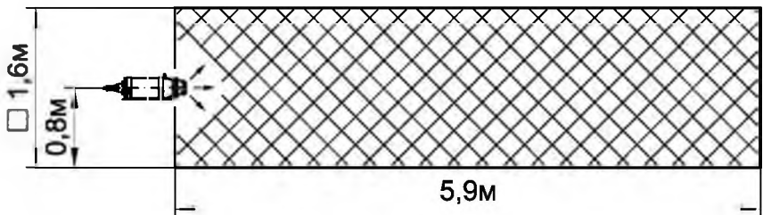
Рисунок 9 - Масштабное изображение области, в которой достигаются условия тушения модулем Буран-2,0(1к) по очагам классов В и А
