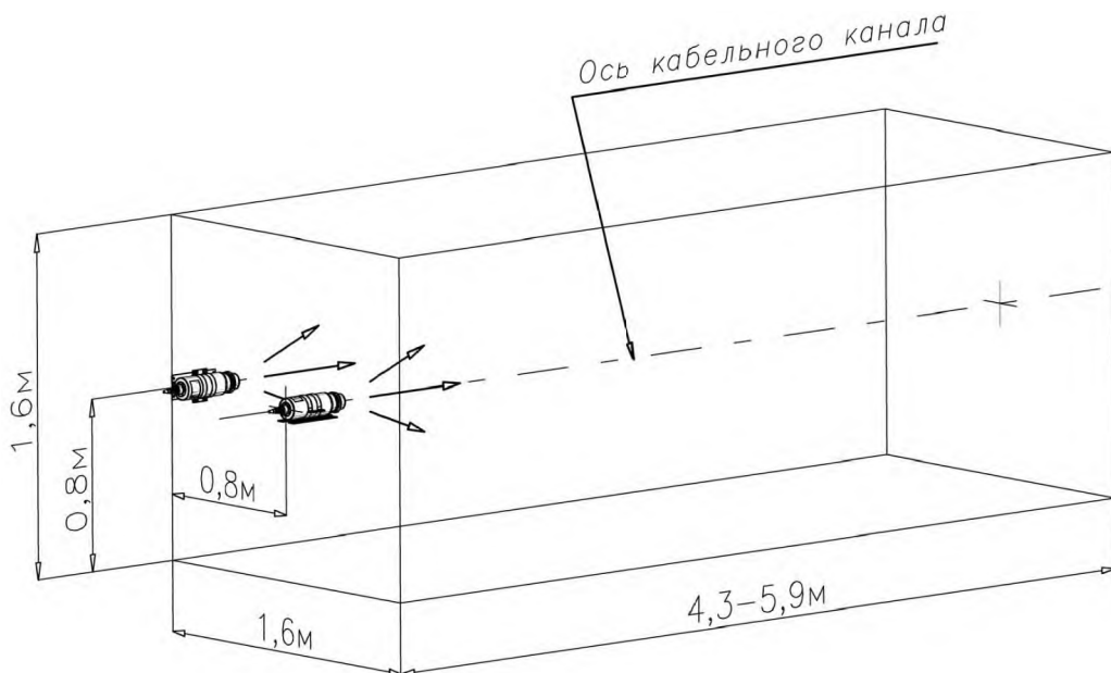
Рисунок 6 - Размещение модулей Буран-2,0(1к) в кабельных каналах или подобных помещениях
