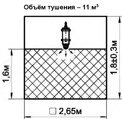
Рисунок 7 - Масштабное изображение области, в которой достигаются условия тушения модулем Буран-2,0(1) по очагам класса В.
