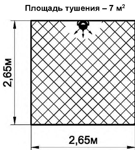
Рисунок 7 - Масштабное изображение области, в которой достигаются условия тушения модулем Буран-2,0(1) по очагам класса В.
