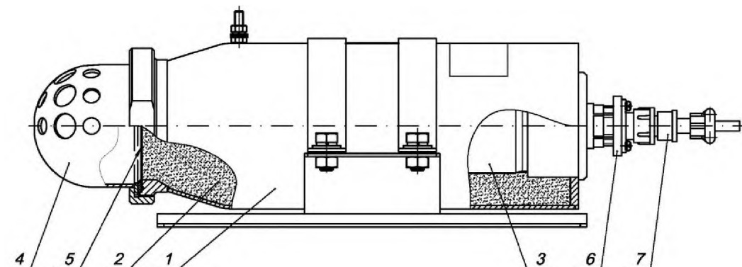
Рисунок 3 - Устройство модуля Буран-2,0
