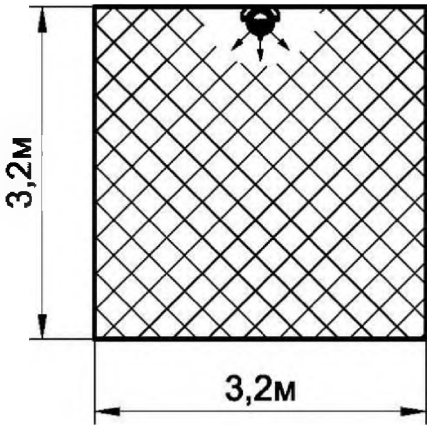
Рисунок 8 - Масштабное изображение области, в которой достигаются условия тушения модулем Буран-2,0(1) по очагам класса А.
